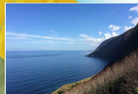
Ponta Furada Ponta Furada
